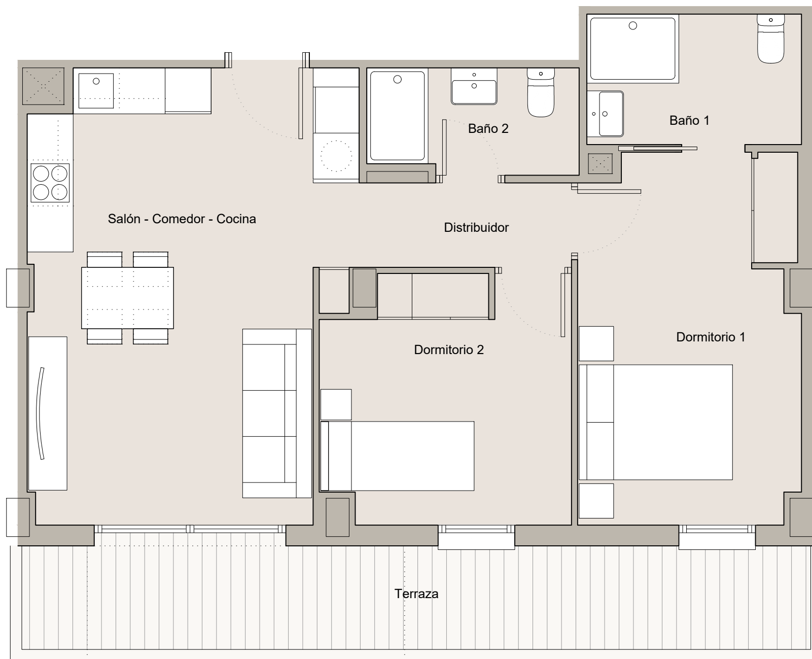
VIVIENDA VT09 ( ACCESIBLE, 2 DORMITORIOS)
