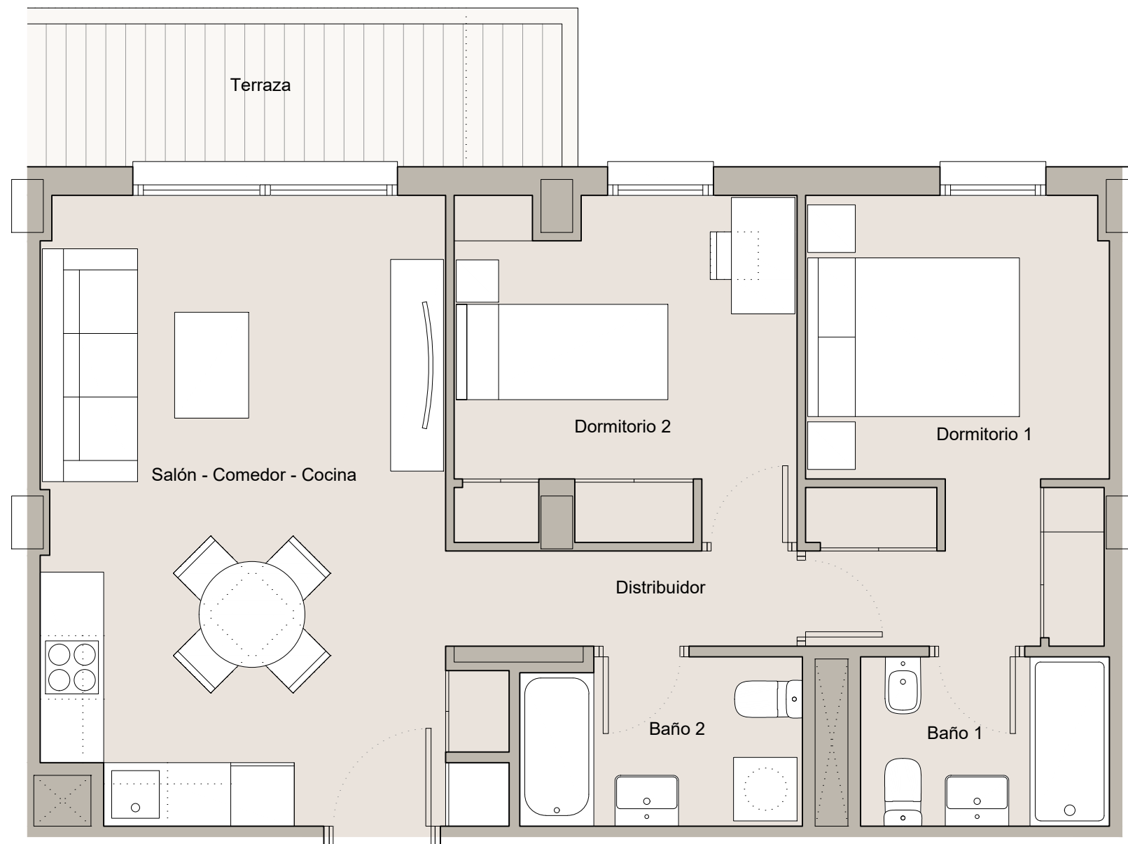
VIVIENDA VT07 ( 2 DORMITORIOS)
