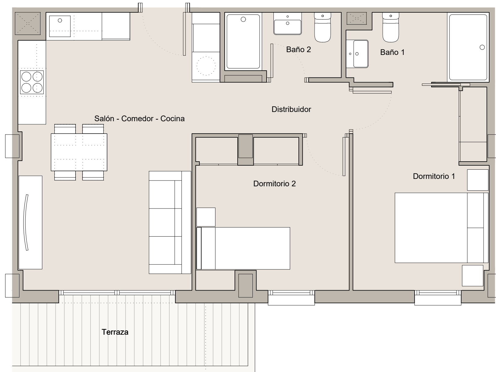
VIVIENDA VT06 ( ACCESIBLE, 2 DORMITORIOS)
