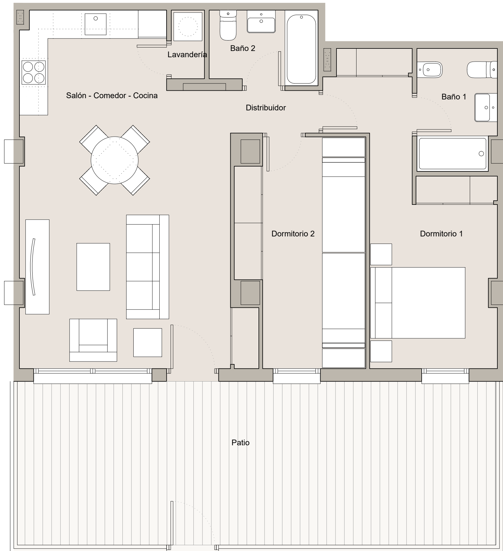
VIVIENDA VT02 (2 DORMITORIOS)
