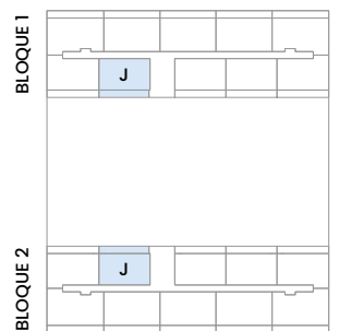
PLANTA PRIMERA
