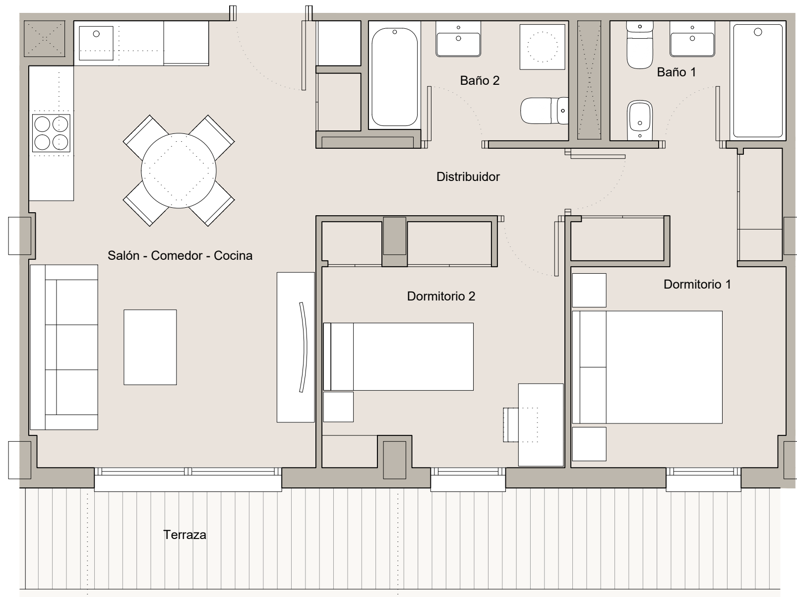
VIVIENDA VT08 ( 2 DORMITORIOS)
