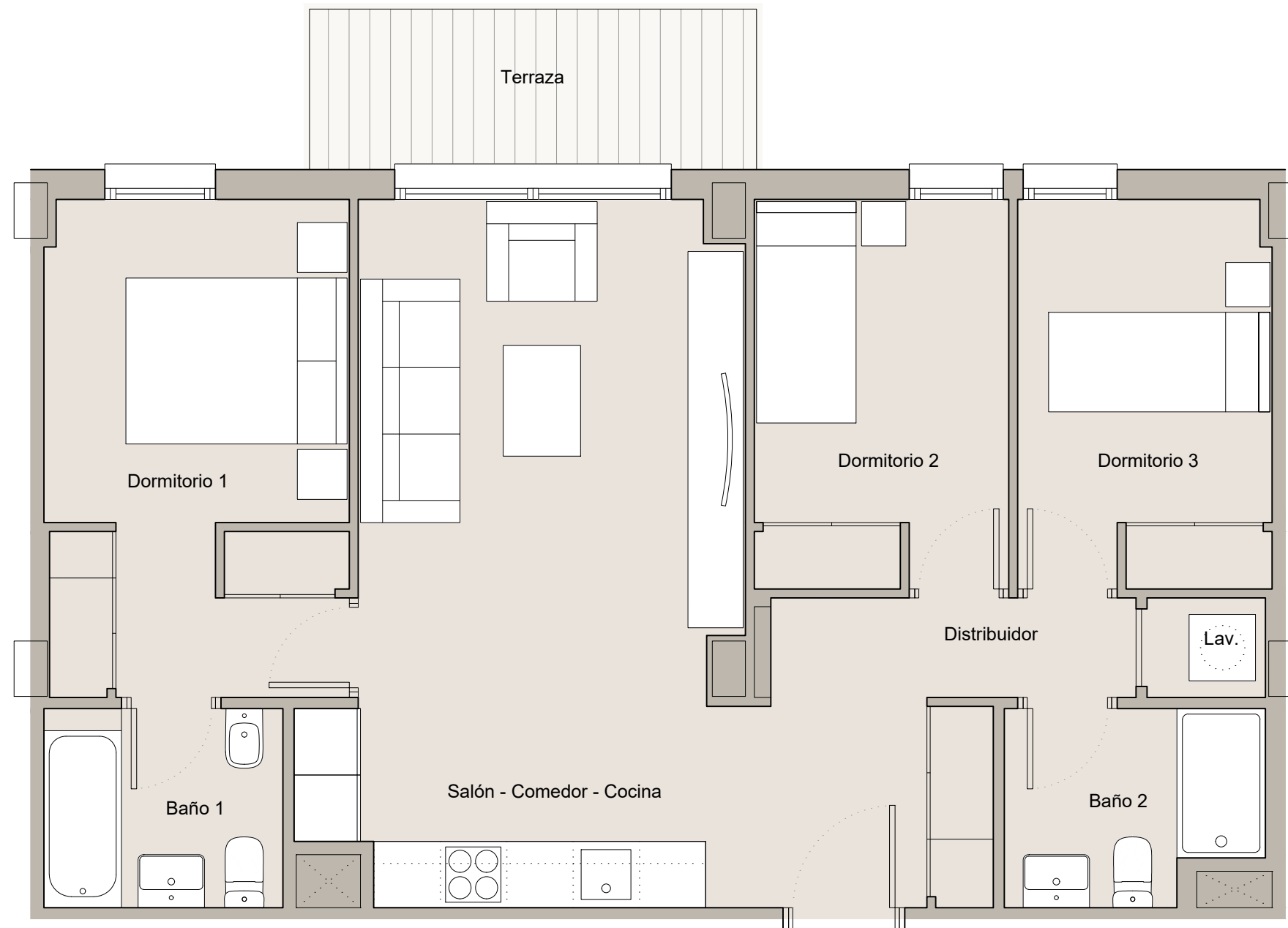
VIVIENDA VT13 ( 3 DORMITORIOS)
