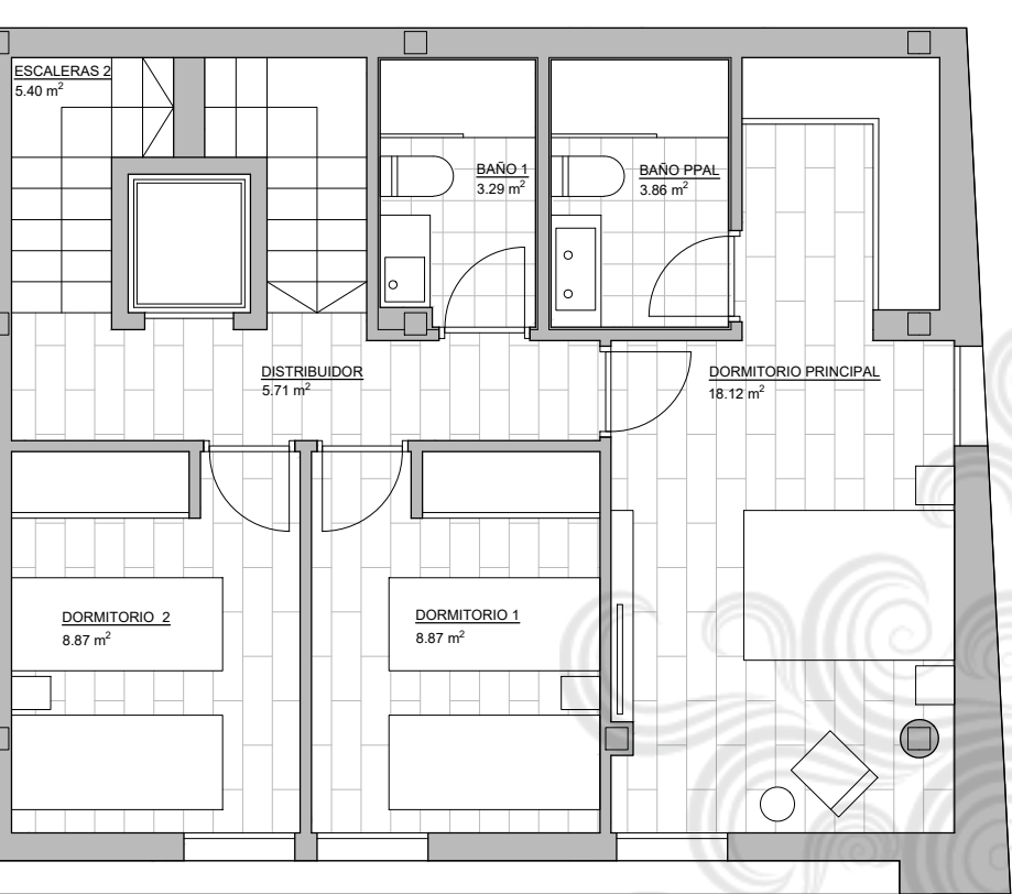
Planta primera
