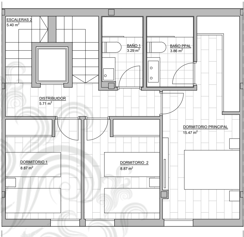
Planta primera
