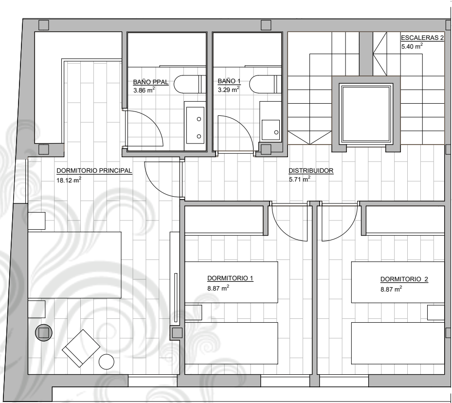
Planta primera
