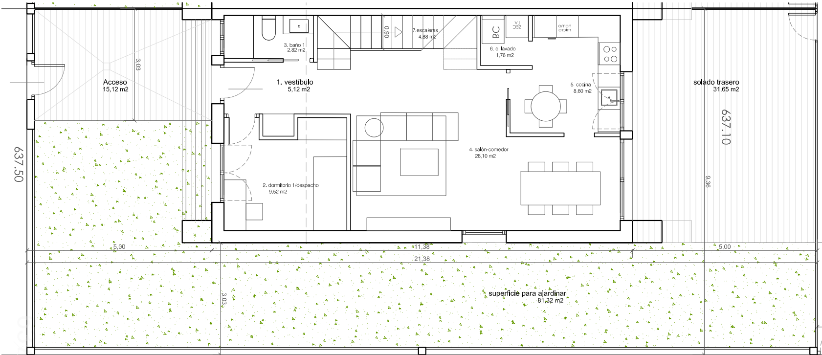
PLANTA BAJA
