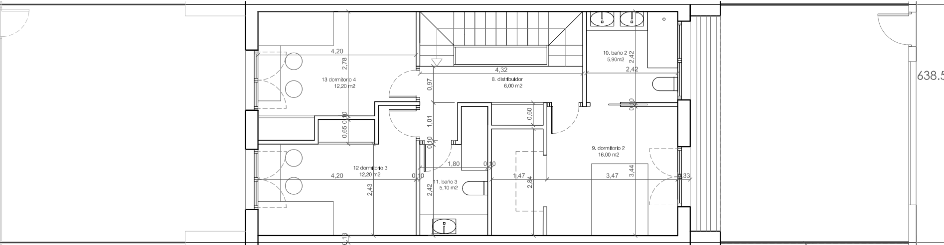
PLANTA PRIMERA
