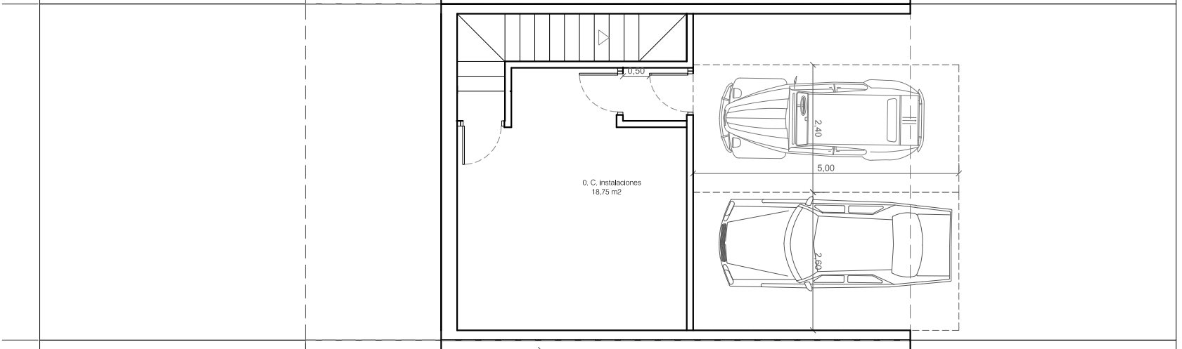
PLANTA SOTANO
