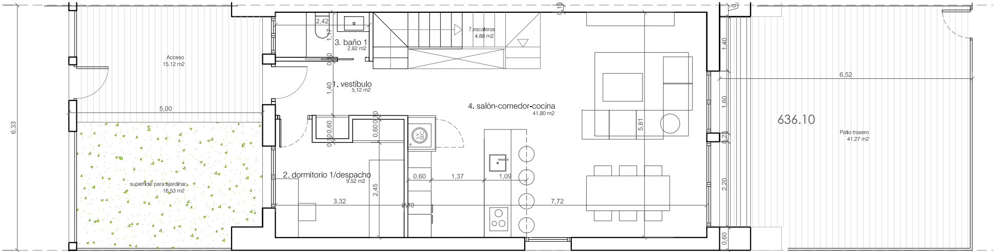
PLANTA BAJA
