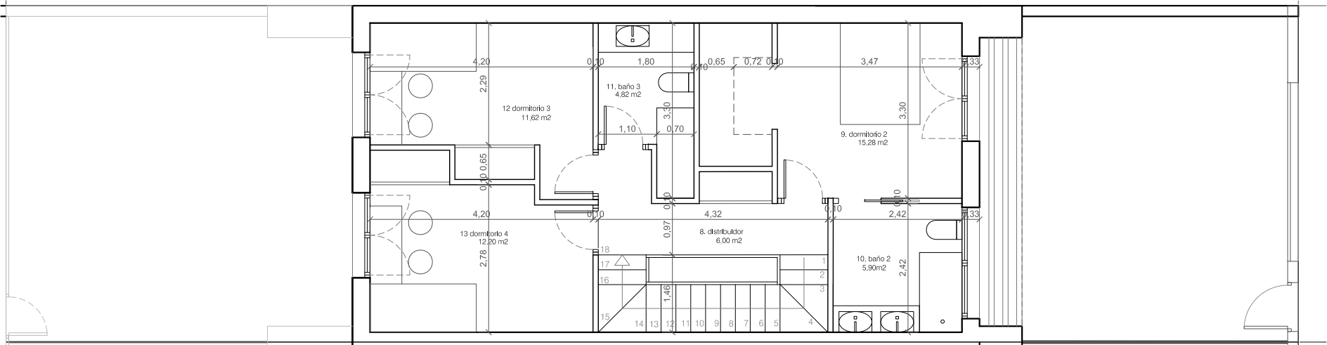
PLANTA PRIMERA
