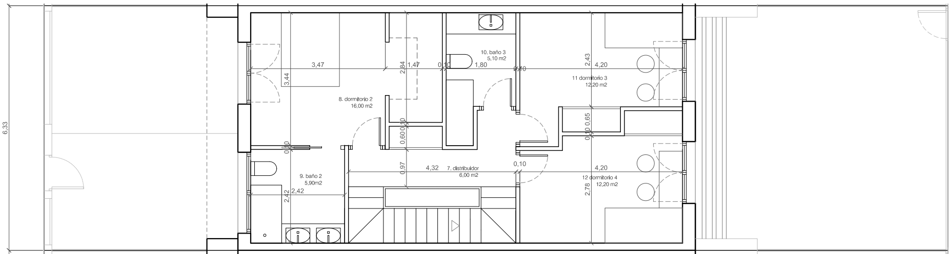
PLANTA PRIMERA
