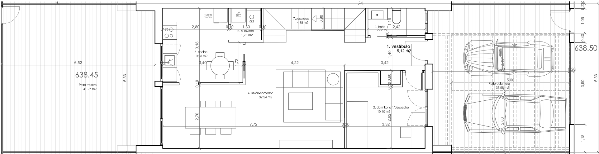
PLANTA BAJA
