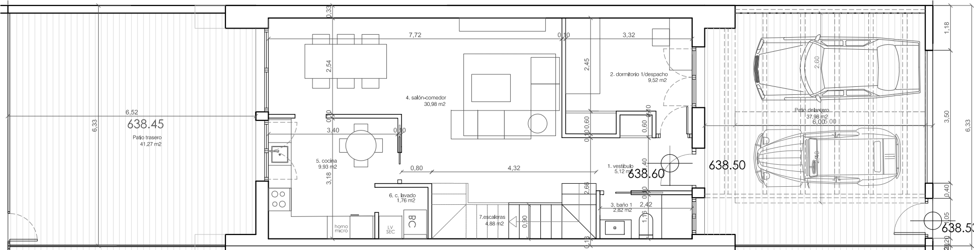
PLANTA BAJA
